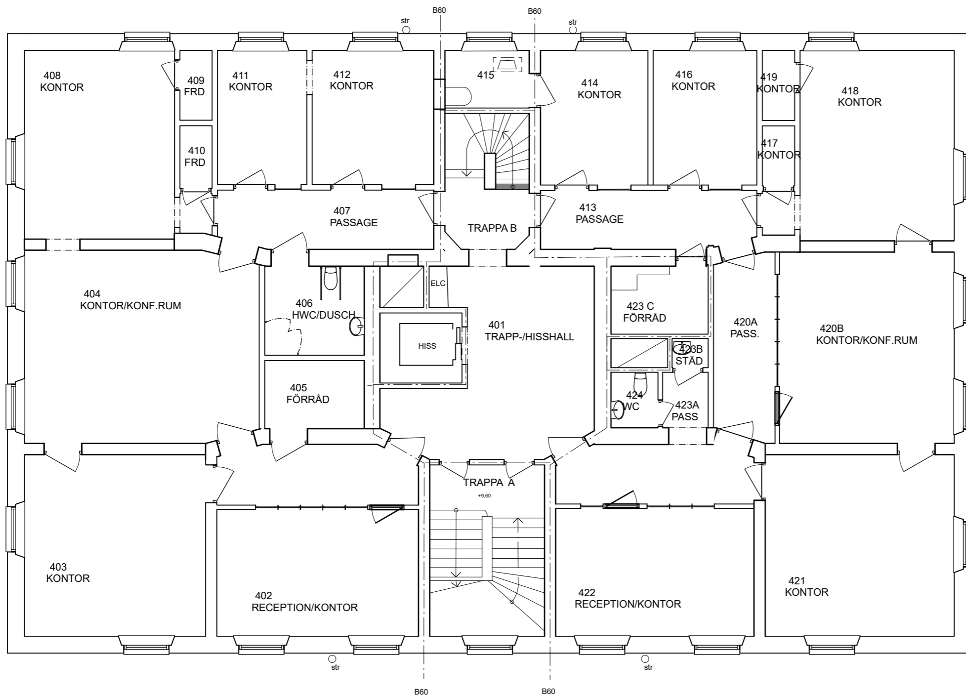
Plan 4 1:100
